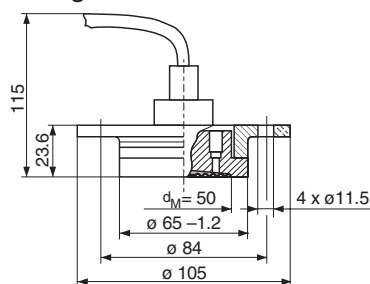
DRD Flange PN 25
