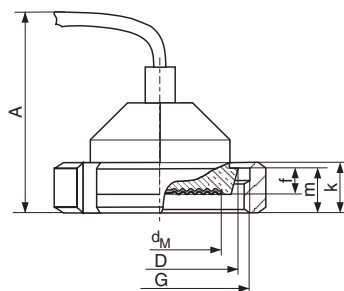
DRD Flange PN 25
