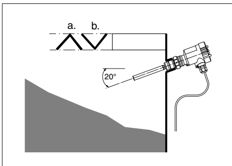
Fig. 18: Montage horizontal
