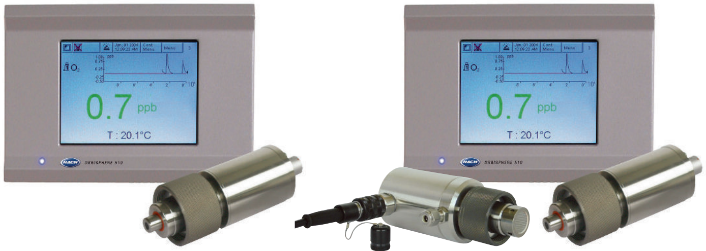
511 Monochannel System (O 2 )
